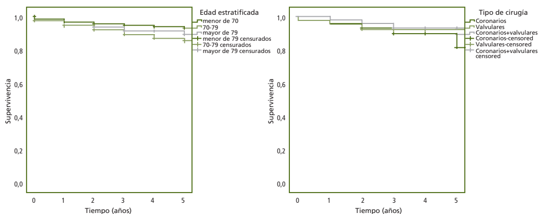
Gràfic 7 | Corba de supervivència després de cirurgia cardíaca a l'HUSE. A, per edat. B, per patologia (en octogenaris)
